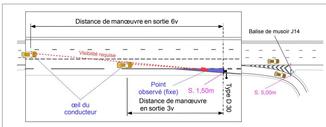
Figure 14 : Visibilité sur sortie en déboîtement ( N_{pv} B )
