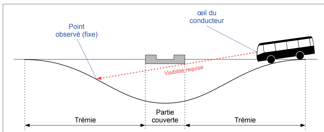
Figure 17 : Visibilité sous ouvrage
