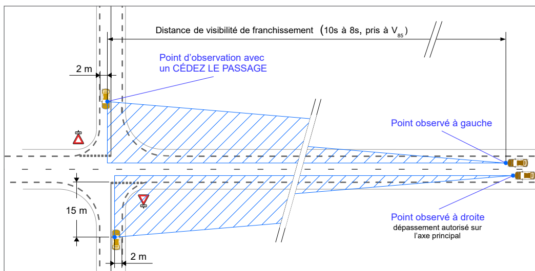
Figure 6 : Construction des triangles de visibilité pour les usagers de la route secondaire - Situation de cédez le passage
